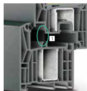
1 Středové těsnění
