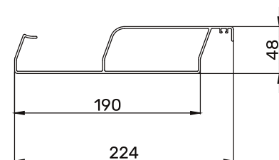
STŘEŠNÍ LAMELA
